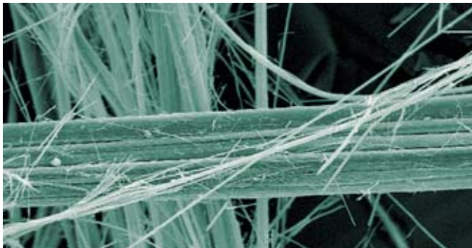
Asbestfasern 1/10 mm
